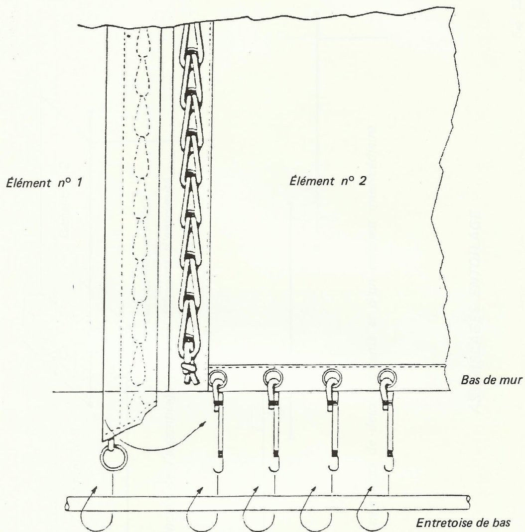
ASSEMBLAGE DES ÉLÉMENTS PAR LAMBIASSAGE ET ACCROCHAGE SUR ENTRETOISE DE BAS
