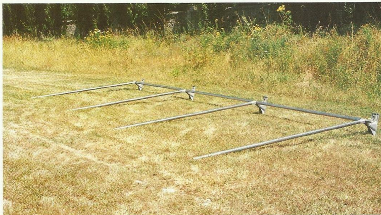
Fig. 14 - Vue de l'armature comportant les 4 semelles, les 3 entretoises et les 4 poteaux
