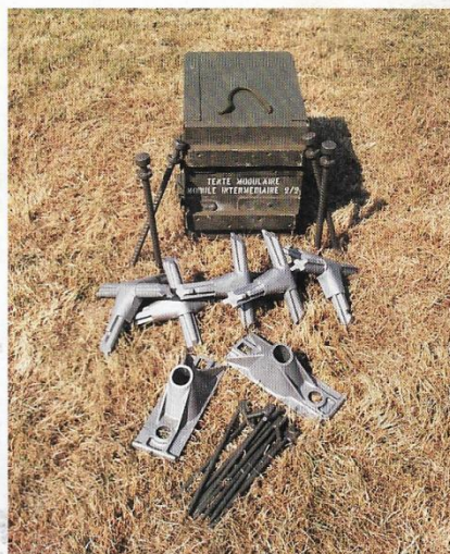
Fig. 10 Caisse d'éléments d'armature et d'accessoires d'un élément intermédiaire
