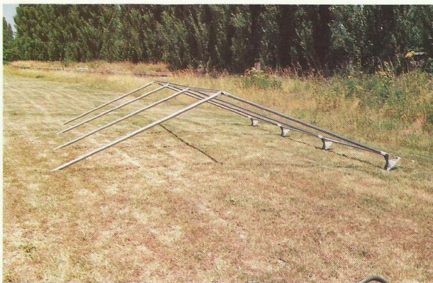
Fig. 15 - Vue d'ensemble de l'armature comportant les semelles, les poteaux, les sablières et les arbalétriers
