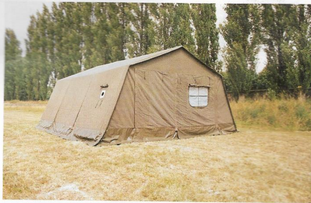
Fig. 1 - Vue d'ensemble de la tente 3 travées
