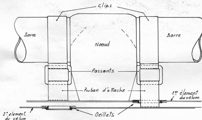
Fig. 26 - Raccordement de deux éléments de vélum
