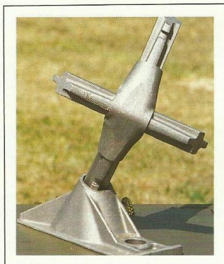
Fig. 12 - Montage d'un nœud sur une semelle Présentation du nœud
