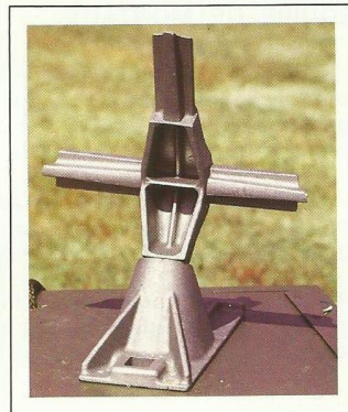
Fig. 13 - Vue du nœud monté sur la semelle
