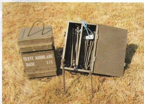
Fig. 7 - Vue de la caisse d'accessoires base 3/3 (fermée et ouverte)
